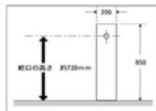
◎ルミエーラ水栓柱が高い場合
